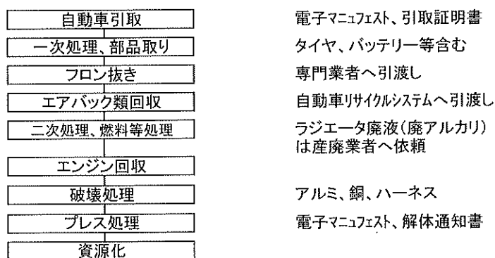
図2 自動車解体フロー
